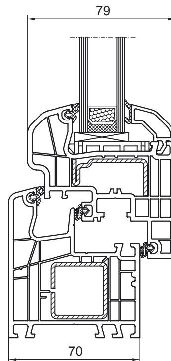
Zugrundeliegende Profil-Kombination
